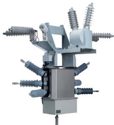
Accionamiento motorizado o manual por transmisión hasta 36 kV (Cat 404)
